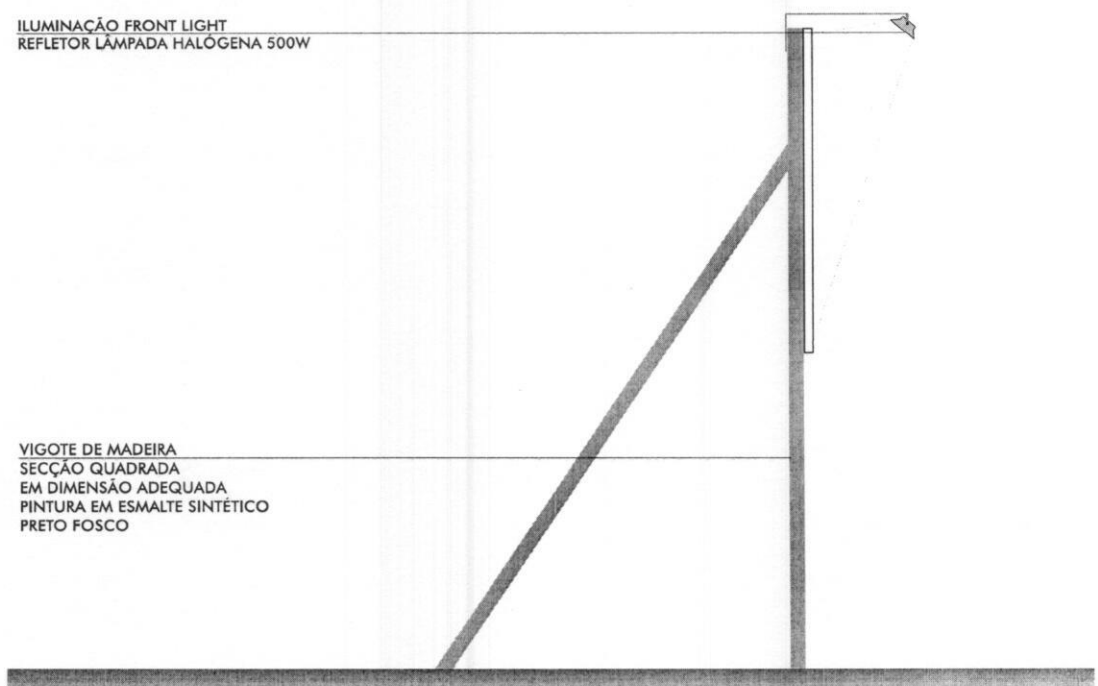
VISTA LATERAL
