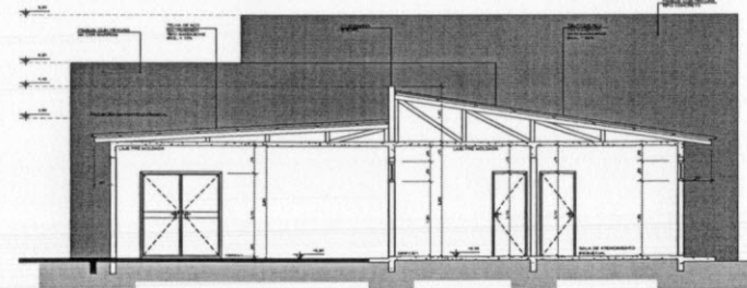
CORTE D-D escala 1:50
