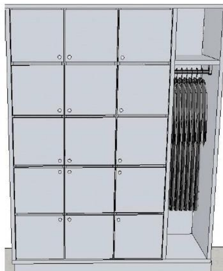
Figura 3PEÇA 02 ARMÁRIO C/15PORTAS C/ CHAVES INDIVIDUAL C/NICHO CABIDEIRO LARG.1.65 ALT.2.10 PROF.0.52 100% MDF 15mm ARAUCO CINZA CRISTAL COM ACABAMENTO 30mm DOBRADIÇAS HD 35mm CABIDEIRO PERFINOBRE QUANTIDADE 01
