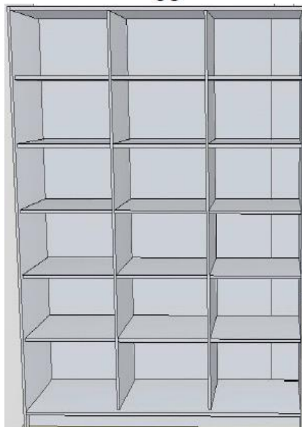
PEÇA 09: ARMÁRIO PRATELEIRAS SEM PORTAS LARG. 2.10 ALT. 2.10 PROF. 0.52 100% MDF ARAUCO CINZA CRISTAL 15mm QUANTIDADE 01
