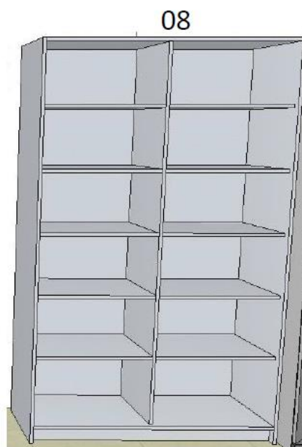
PEÇA 08: ARMÁRIO PRATELEIRAS S/PORTAS LARG. 1.35 ALT. 2.10 PROF. 0.52 100% MDF ARAUCO CINZA CRISTAL 15mm QUANTIDADE 01
