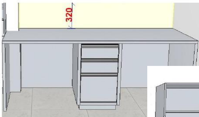
PEÇA 06: MESA ESCRITÓRIO C/03 GAVETAS SENDO UMA FIXA MDF DE 30mm 100% MDF ARAUCO CINZA CRISTAL PUXAD PERFINOBRE E DOBRADIÇAS HD 35mm 100% MDF LARG. 2.1 0.70 QUANTIDADE 01
