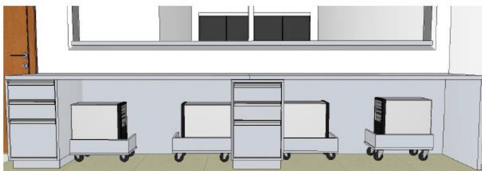
Figura 1 PEÇA 10: MESA E BANCADA RECEPÇÃO COM 06 GAVETAS SENDO 02 C/FICHÁRIO E 04 SUPORTES "CPU" C/RODÍZIOS PUXADORES GOLF PERFINOBRE CORRIDIÇAS RODÍZIOS HD TAMPO E PÉS MDF DE 30mm QUANTIDADE 01
