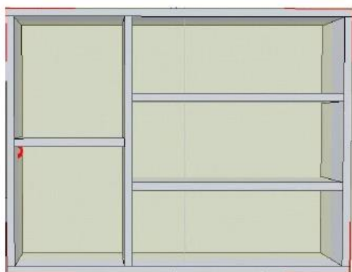
PEÇA 07: PRATELEIRA 100% MDF ARAUCO CINZA CRISTAL DE 30mm C/ FUNDO LARG. 1.29 ALT. 1.00 PROF. 0.30 QUANTIDADE 01
